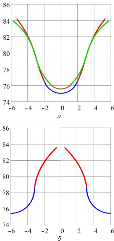
Рис. 1 – Профили синтезированных зубьев: a – сопряженная пара зубьев зубчатой передачи с параметрами – m=4\text{мм} , \alpha_0=15^\circ , z_1=20 , z_2=40 , k=-5 ; b – зуб звездочки цепной передачи с параметрами – шаг цепи t=25,4\text{мм} , z=20 , k=-5
