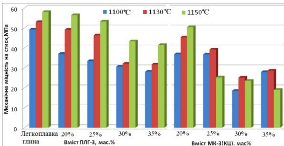
Рис. 4 – Залежність: а – водопоглинання, б – механічної міцності на стиск від складу керамічних мас для зразків, випалених при різних температурах.
