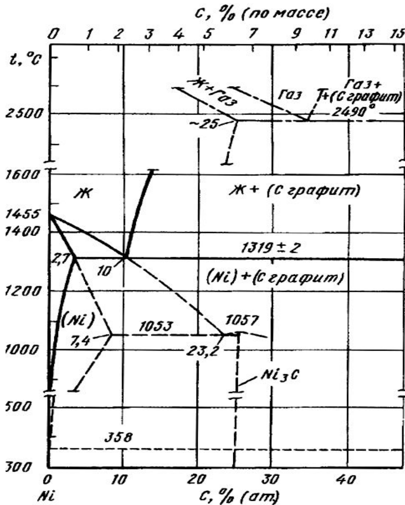
Рис. 3 – Діаграма стану системи Ni – C
