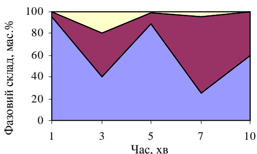
Рис. 3. – Зміна фазового складу осадів карбонату кальцію при 363 К: \square кальцит; \blacksquare арагоніт; \blacksquare ватерит.
