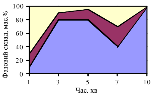
Рис. 2. – Зміна фазового складу осадів карбонату кальцію при 343 К: \square кальцит; \blacksquare арагоніт; \blacksquare ватерит.
