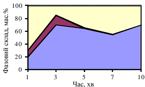
Рис. 1. – Зміна фазового складу осадів карбонату кальцію при 323 К: \square кальцит; \blacksquare арагоніт; \blacksquare ватерит.
