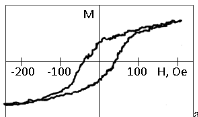
Рисунок 2 – Петлі гістерезису покриття Fe-Co-Mo за тривалості електролізу: а – 1 хв, б – 10 хв
