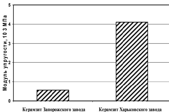
Рис. 1. Прочностные и упругие свойства керамзита
