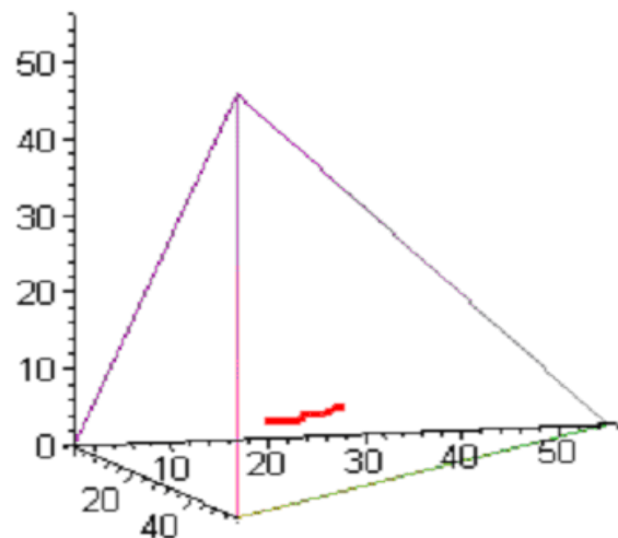
Рис. 5. Решение задачи
