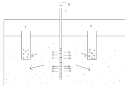
Рис. 1. Схема подачи нейтрализатора через напорную скважину в зону загрязнения (по бокам расположены приемные коллектора)
