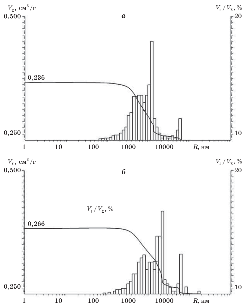
Рис. 5. Результаты ртутной порометрии: а — образец без добавки, б — образец с 2 % добавки
