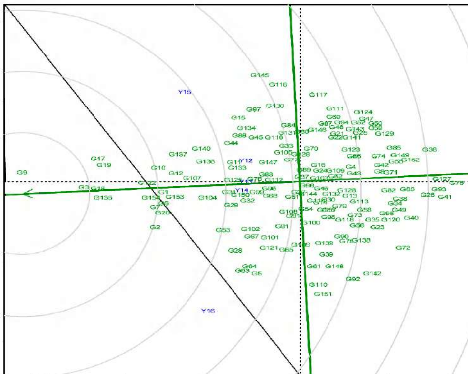
Рис. 4. Ранжирування селекційних ліній ячменю озимого по відношенню до гіпотетичного «ідеального» генотипу, 2012-2016 рр.
