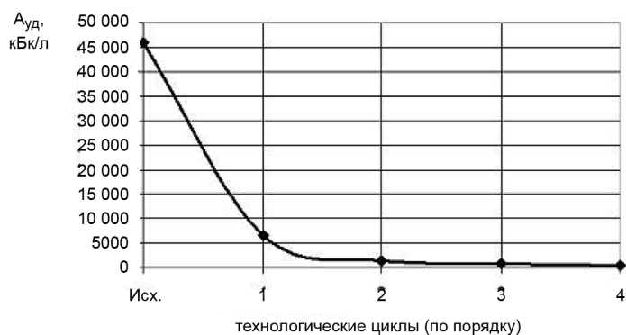
Рис. 1. Сорбция радионуклидов из водных растворов, содержащих ^{90}\text{Sr}
