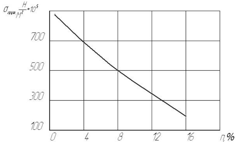
Рисунок 1 – Залежність міцності склопластику ( \sigma_{зруш.} ) від вмісту порожнин у структурі (n) [17]
