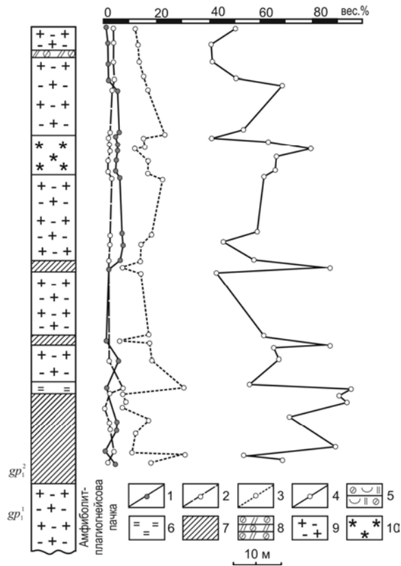
Рис. 6. Характер изменения порообразующих окислов в амфиболит-гнейсовой пачке северо-восточного крыла Гуляйпольской синклинали: 1-4 вариации содержания окислов по направлению истинной мощности пачки: 1 – Na, 2 – K, 3 – Al, 4 – Si; 5-10 – породы: кварц-гранат-биотитовые сланцы – маркирующий горизонт (5), кварц-мусковитовые сланцы (6), в т.ч. с андалузитом, кианитом, биотитом, ставролитом; алюмокварциты (7); амфиболиты (8); биотит-полевошпатовообманковые гнейсы в различной степени мигматизированные, переходящие вверх по разрезу в двуслюдяные гнейсы одноименной пачки (9); биотит-полевошпатовообманковые гнейсы с магнетитом (10).
